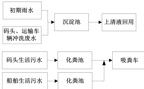
图4-1 废水处理流程图
