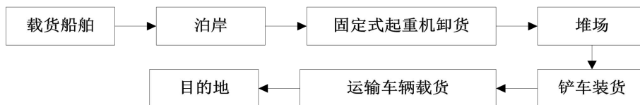
图 3-3 本项目工艺流程图
