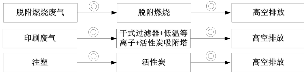
图4-2 废气处理设施流程图 废气治理设施图片：
